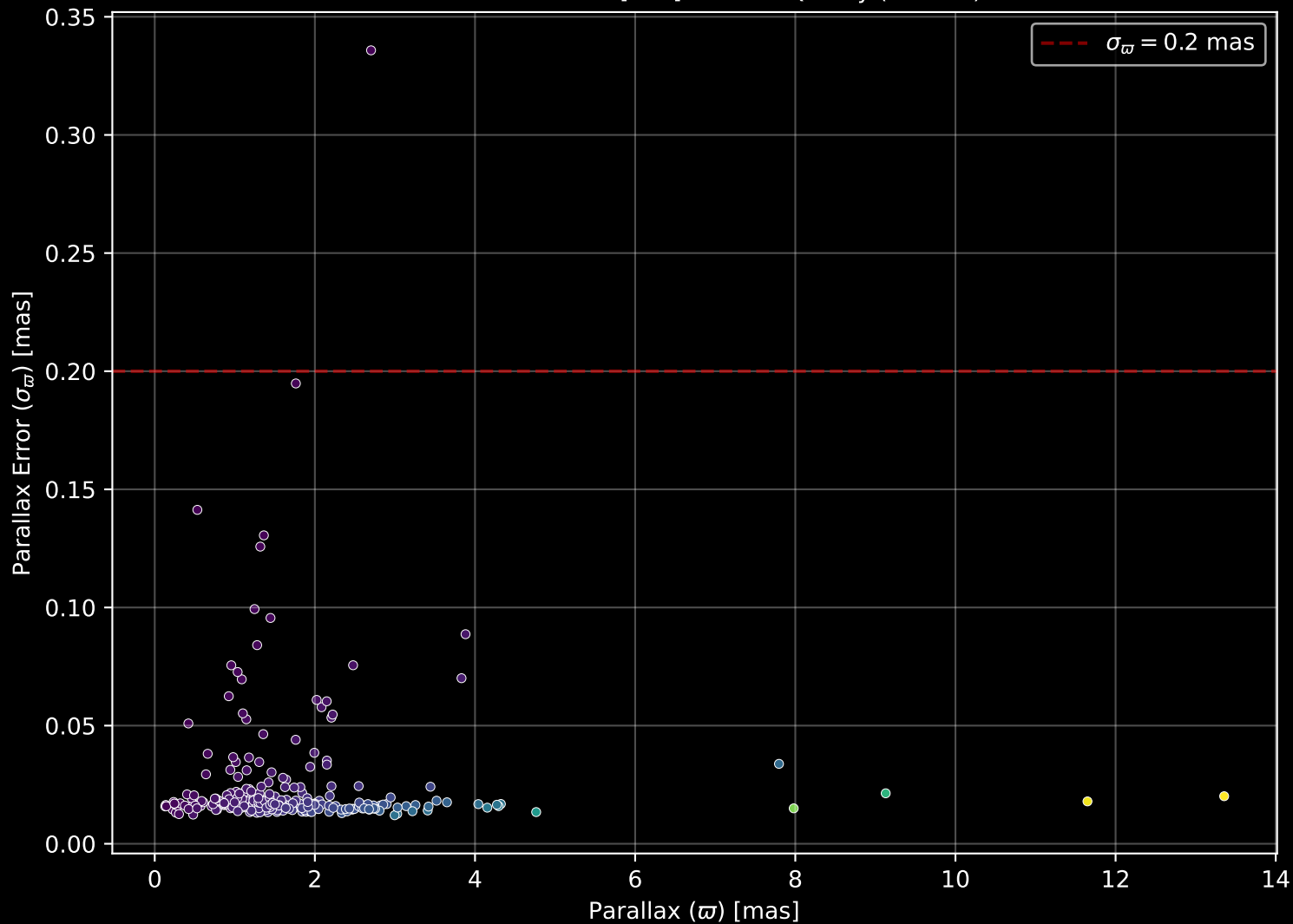
GALAH DR4 Field: [886] Parallax Quality (n= 285)
