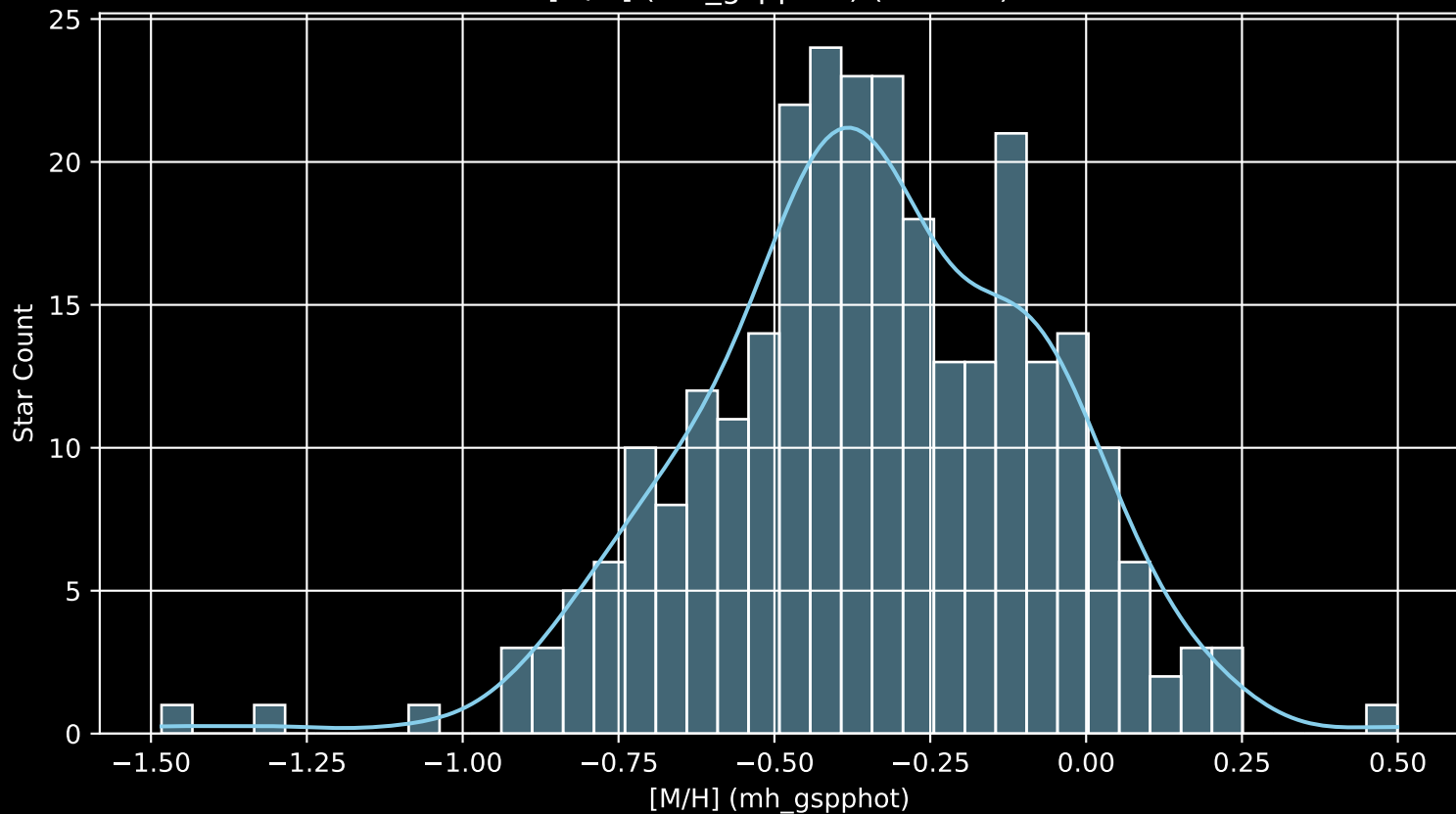
GALAH DR4 Field: [886] [M/H] (mh_gspphot) (n= 284)
