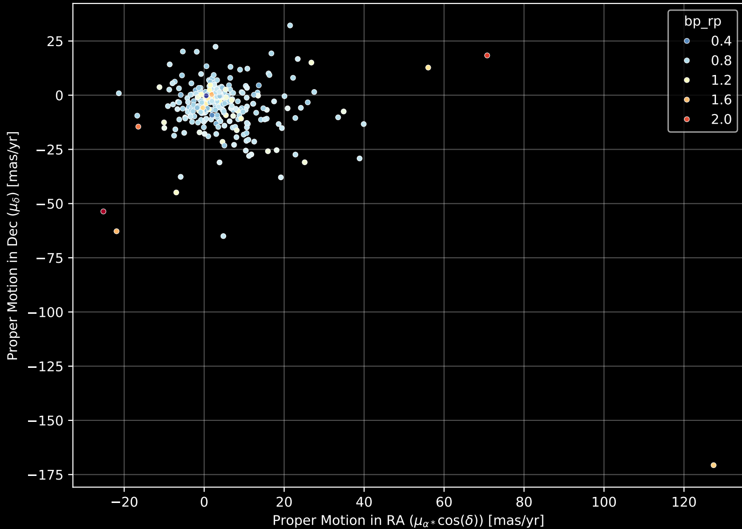
GALAH DR4 Field: [886] Proper Motion Diagram (n= 285)
