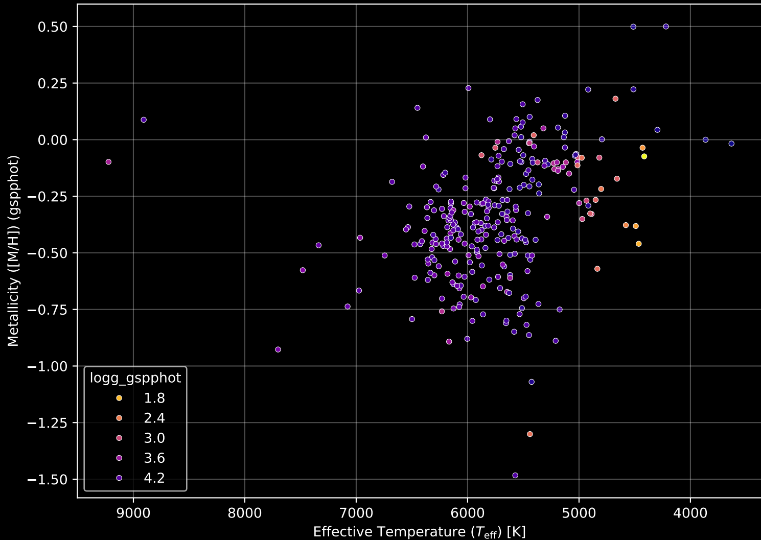
GALAH DR4 Field: [886] Stellar Population Parameters (n= 285)
